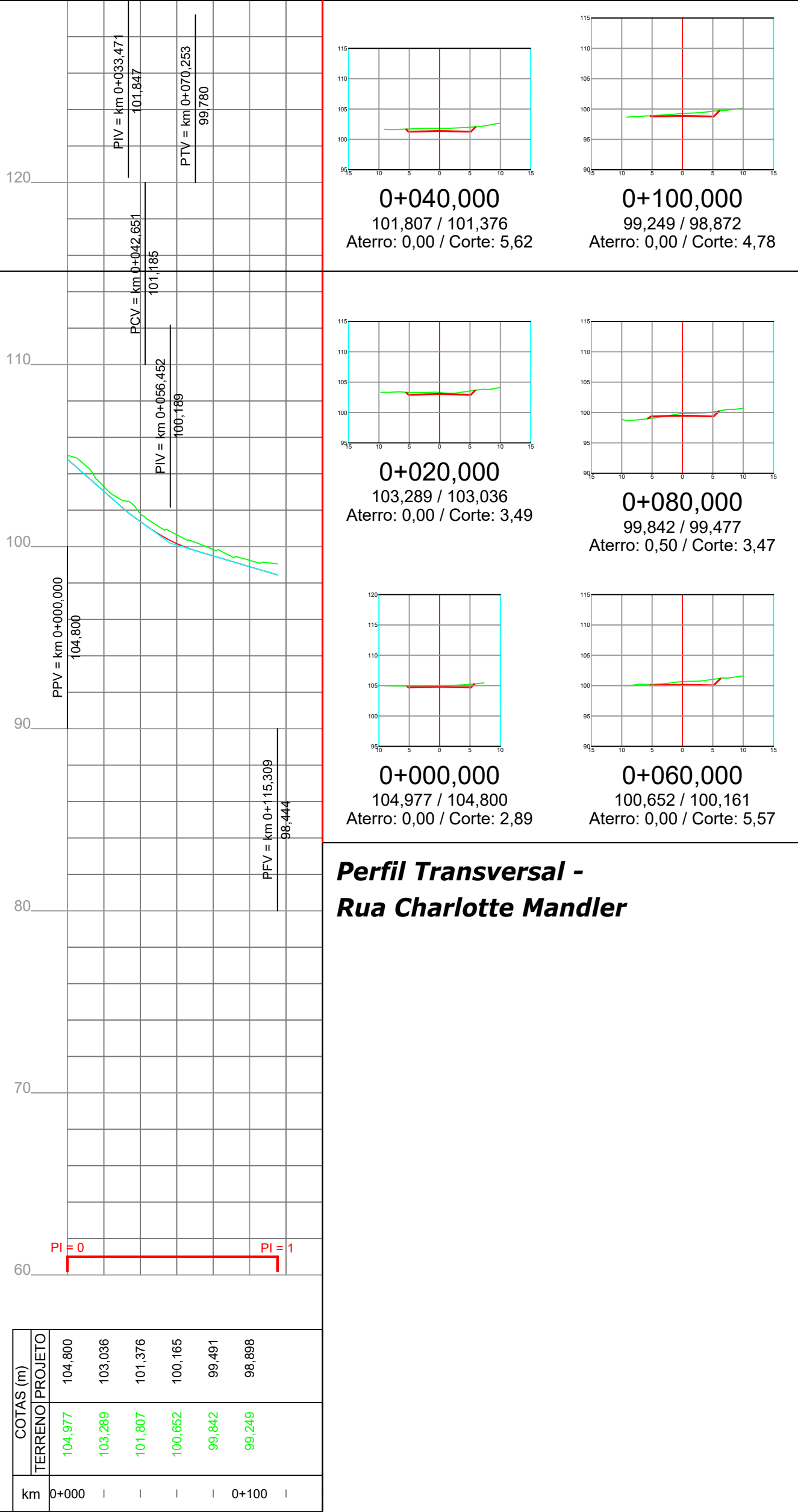
Perfil Longitudinal - Rua Charlotte Mandler Escala: 1/2500
