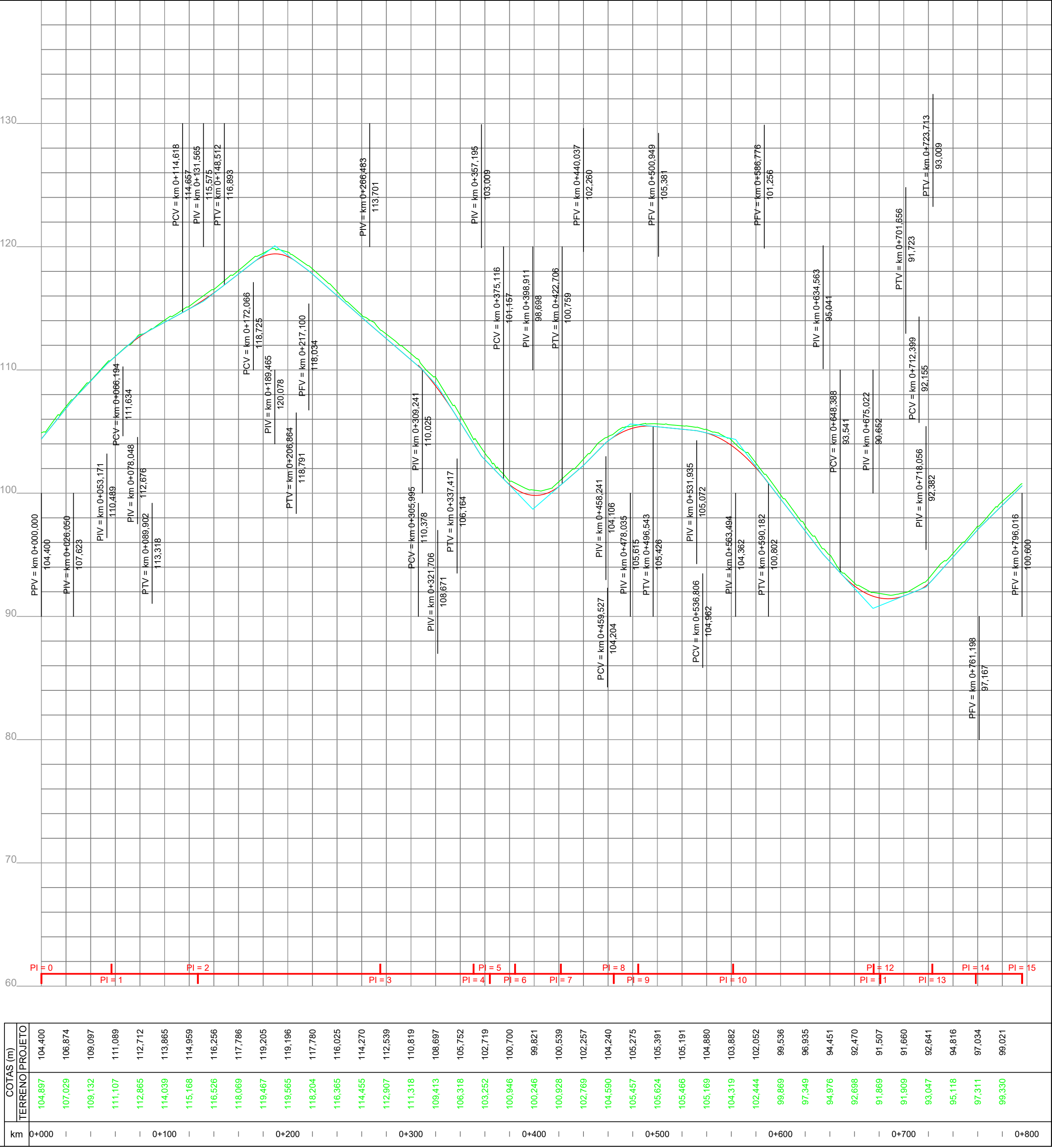
Perfil Longitudinal - Rua José Severino Pick Escala: 1/2500
